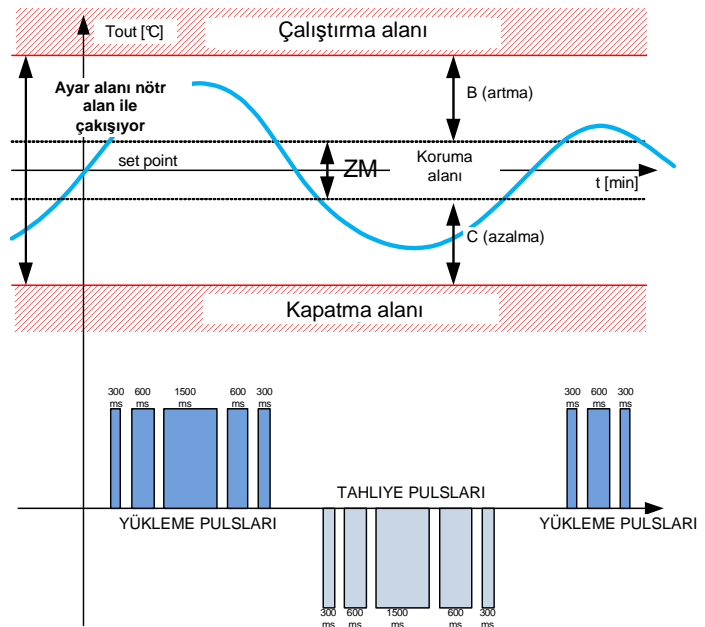
Resim 1.6.4.i: vidalı kompresörler için modülasyon ayarı
