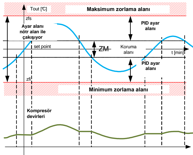
Resim 1.6.5.m: çıkışta PID regülatörü çalışma diyagramı
