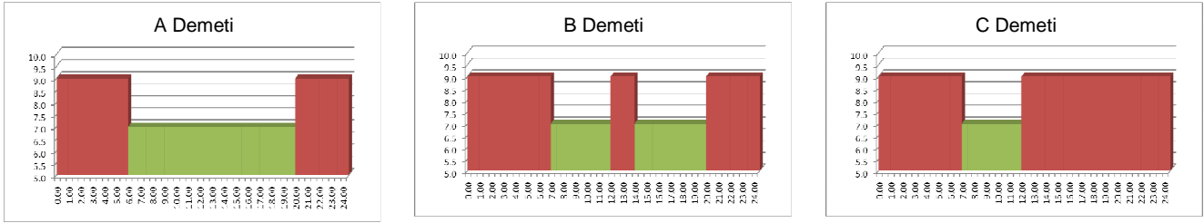
Resim 1.4.a: saat dilimlerinin günlük düzenlenme örnekleri ■ Ayarlama ■ Ünite Kapalı
