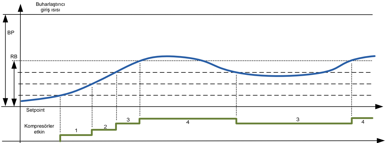
Resim 1.6.5.k: offset = 0 ve Rb = % 50 olacak şekilde giriş sensörü üzerinde esnek kademeli orantılı ayar
