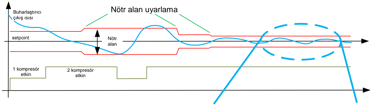
Resim 1.6.6.n: çıkış sensörü üzerinde nötr alanlı ayar
