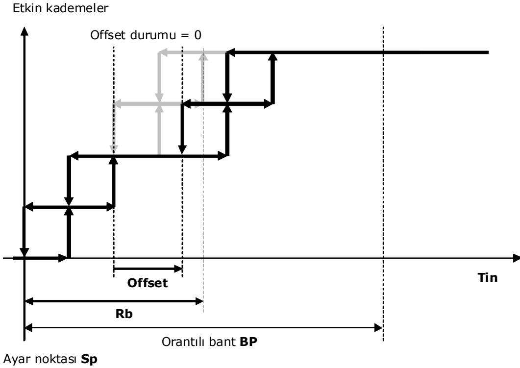
Resim 1.6.5.l: offset > 0 ve Rb = % 50 olacak şekilde kademeli orantı regülatörü
