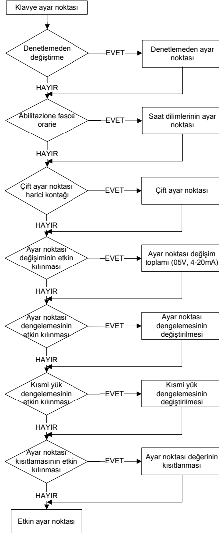
Resim 1.7.a: etkin ayar noktasını elde edinceye kadar düzenlenmiş olan ayar noktasını değiştirme işlevleri sırası.
