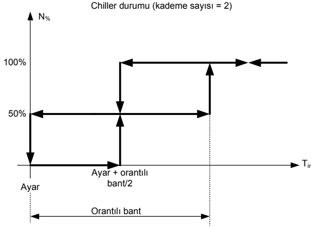
Resim 1.6.1.a: T_{in} giriş değişkenidir, N_{\%} % olarak belirtilmiş etkin kademelerin sayısıdır (chiller durumu)
