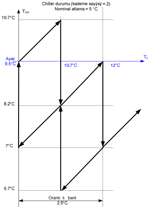
Resim 1.6.1.c: T_{in} ve T_{out} arasında, 2 kademeli ilişki (chiller durumu)
