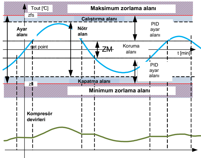
Resim 1.6.6.o: çıkışta PID regülâtörü çalışma diyagramı
