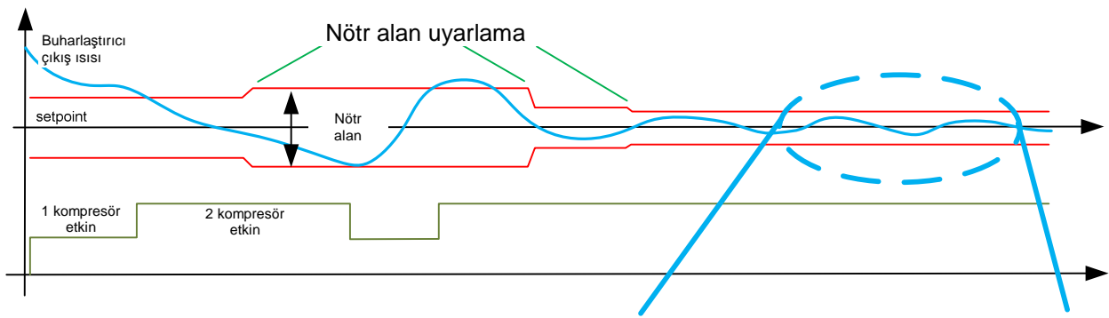
Resim 1.6.4.h: çıkış sensörü üzerinde modülasyon ayarı
