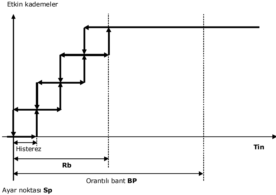
Resim 1.6.5.j: offset = 0 ve Rb = % 50 olacak şekilde kademeli orantı regülatörü
