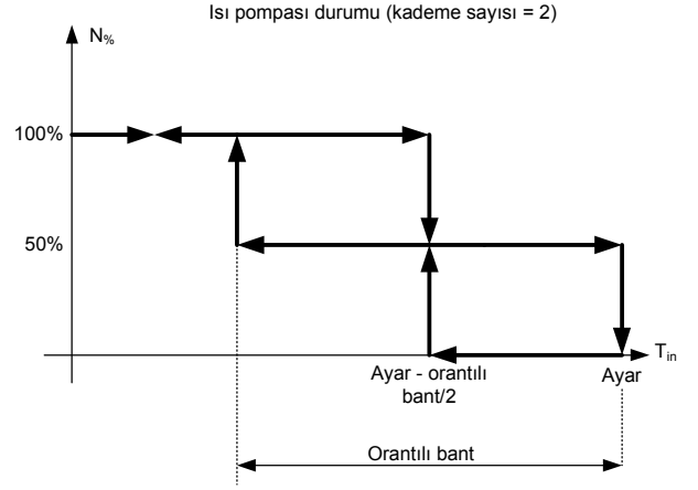
Resim 1.6.1.b: T_{in} giriş değişkenidir, N_{\%} % olarak belirtilmiş etkin kademelerin sayısıdır (ısı pompası durumu)
