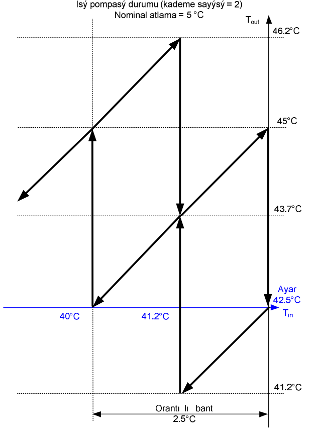
Resim 1.6.1.d: T_{in} ve T_{out} arasında, 2 kademeli ilişki (ısı pompası durumu)
