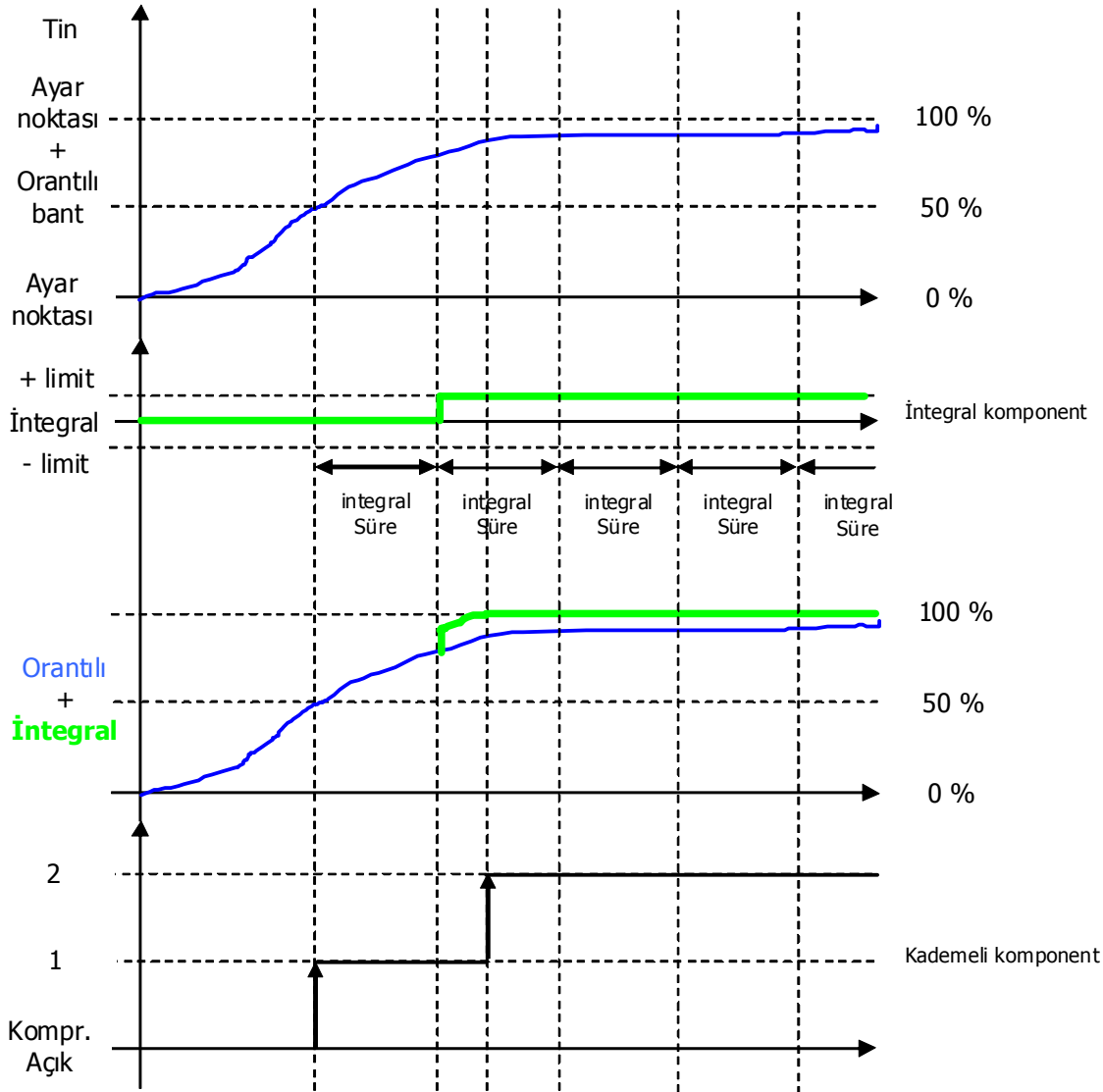
Resim 1.6.2.e: 2 kademeli chiller'de ayar örneği
